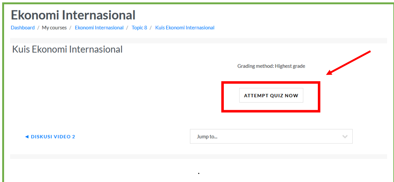
Gambar 2 Halaman kuis
